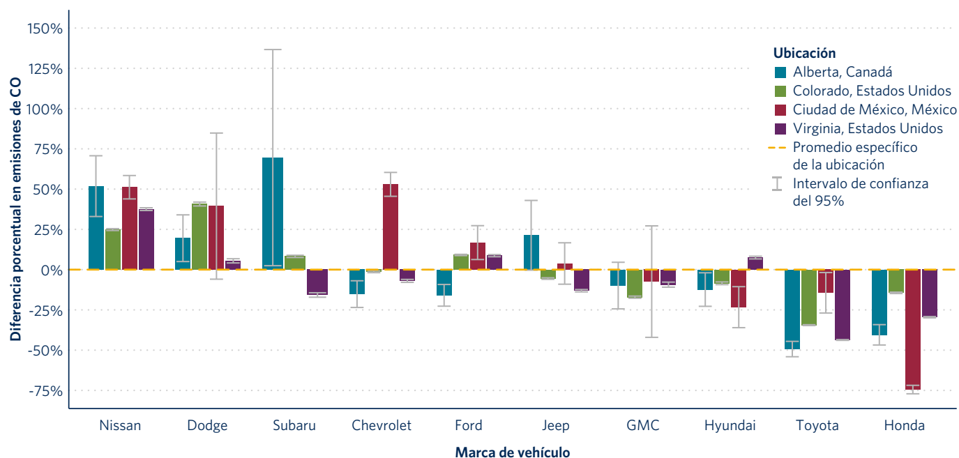
Figura 4. Diferencia en emisiones de CO respecto al promedio específico de la ubicación por marca de vehículo
