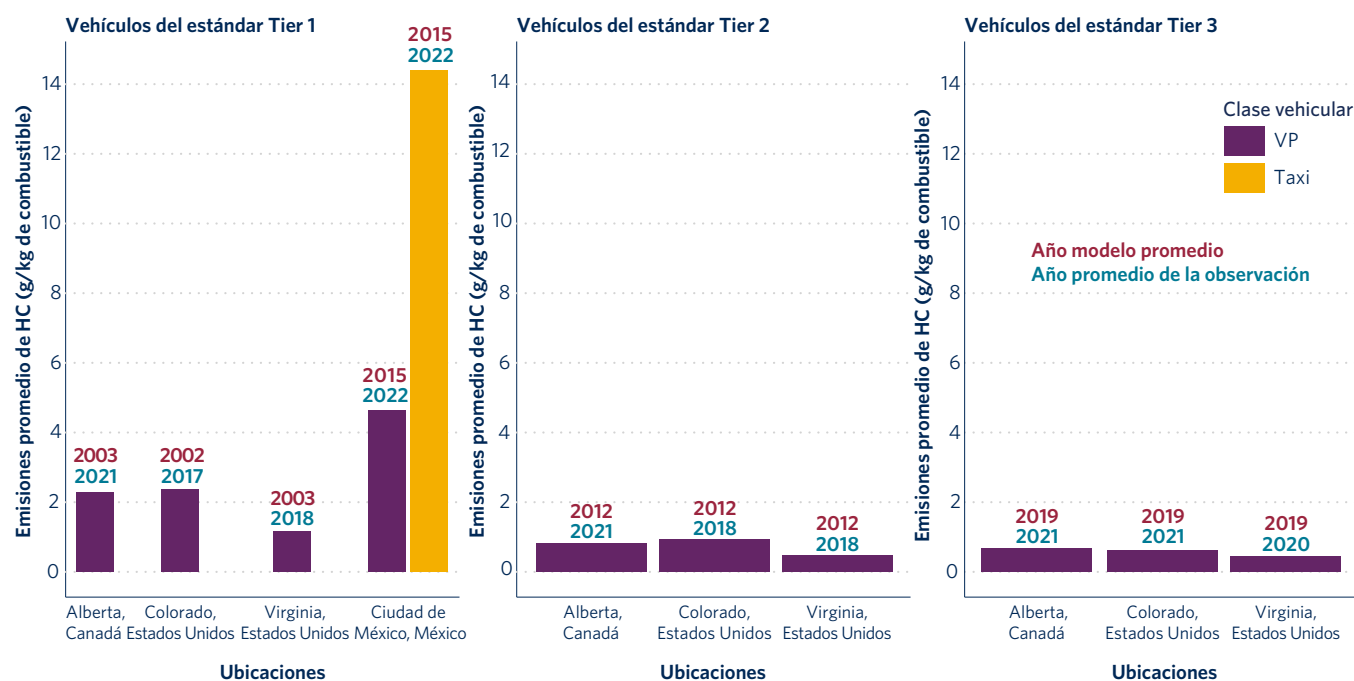
Figura 3. Emisiones promedio de HC por kilogramo de combustible quemado por estándar de emisiones, ubicación y clase vehicular
