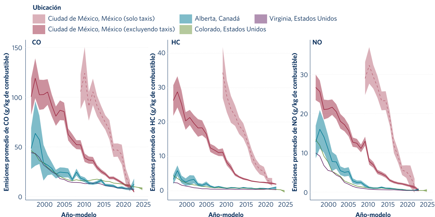
Figura 2. Emisiones promedio por año-modelo para los LDV a gasolina en cada región
